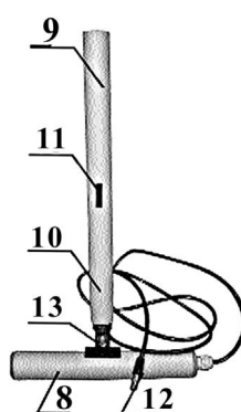
электромагнитный датчик ЭМД-226М
