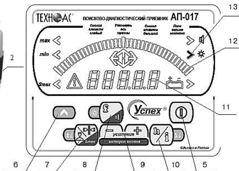
Лицевая панель. Органы управления и индикации
